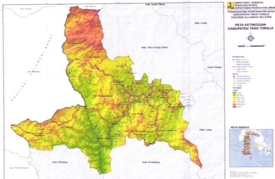
Gambar 2.2 Peta Ketinggian Kabupaten Tana Toraja
