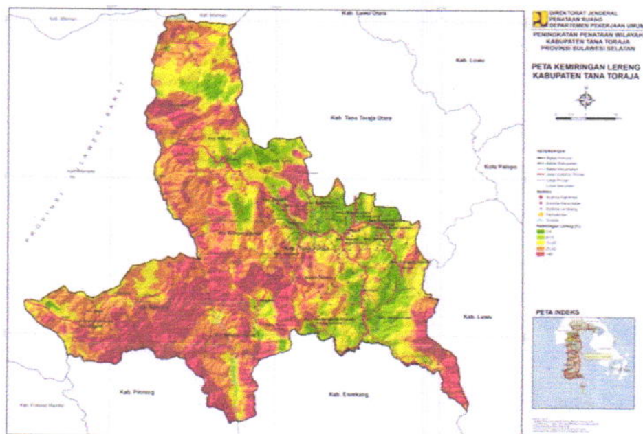
Gambar 2.3 Peta Kemiringan Lereng Kabupaten Tana Toraja
